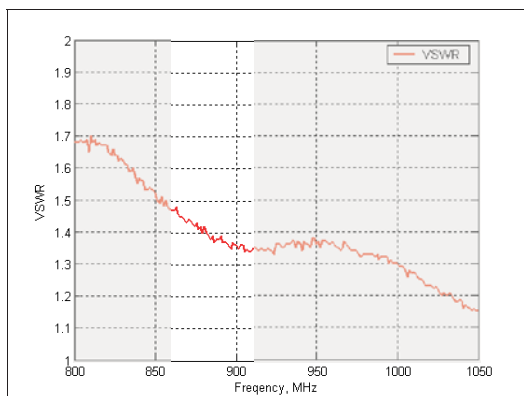
VSWR:
